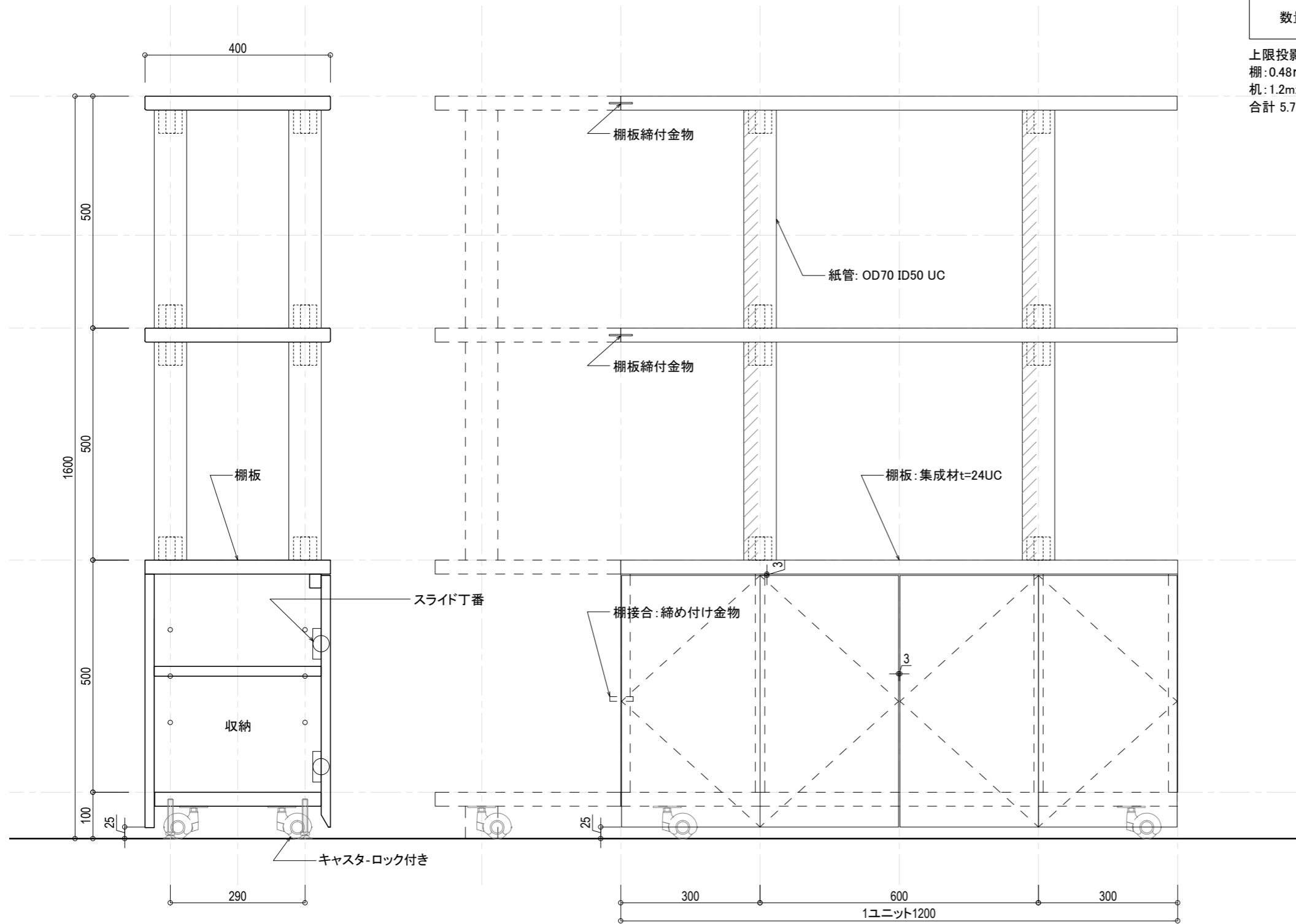
ショップ棚 開き戸ユニット
